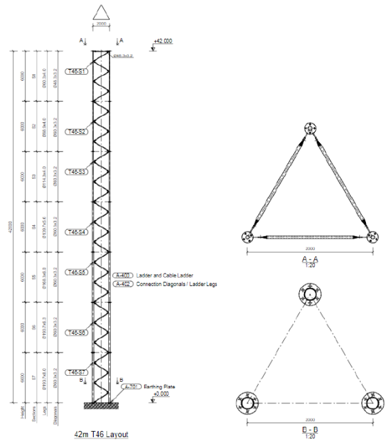
Principtegning af 42m gittermast –
