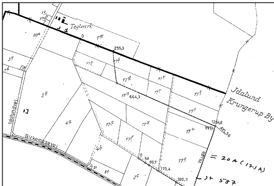
Figur 2 – Kortudsnit fra regulativ for Hanemoseløbet 20A. Ønsket omlægning fra station 255,3 til 664,3.
