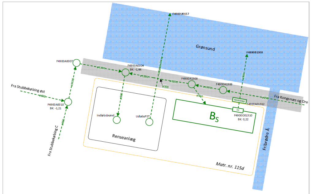
Figur 2 Principskitse over overløbet fra bassinet ved Stubbekøbing Renseanlæg
