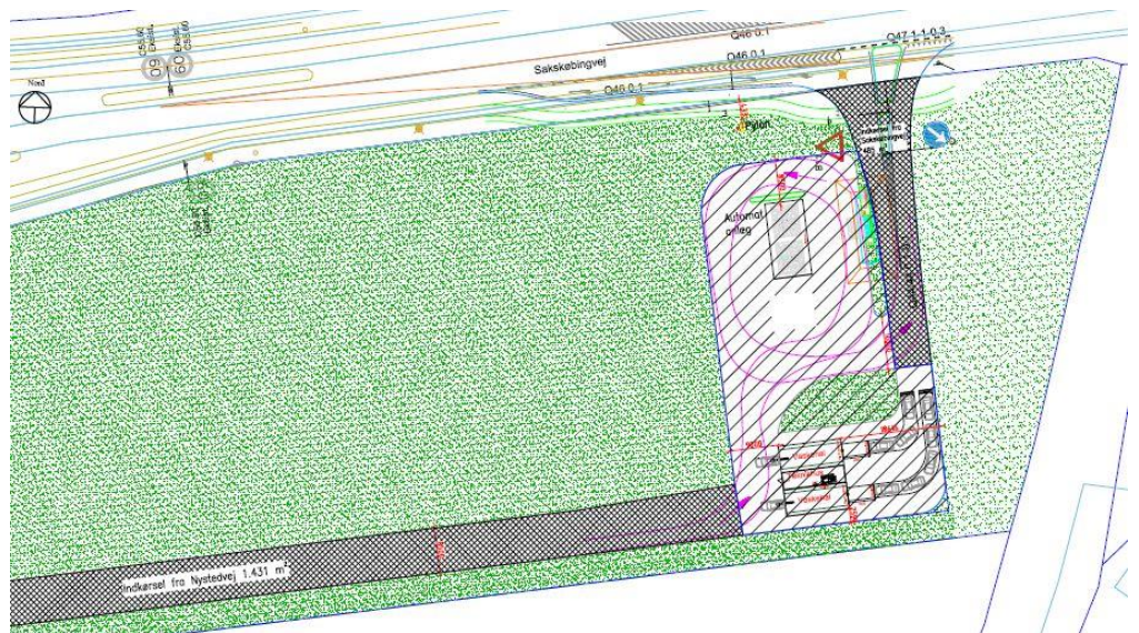
Situationsplan over den ansøgte tankstation med vaskehal
